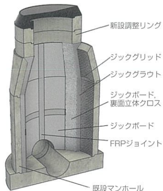
ジックボードJ工法の構成
