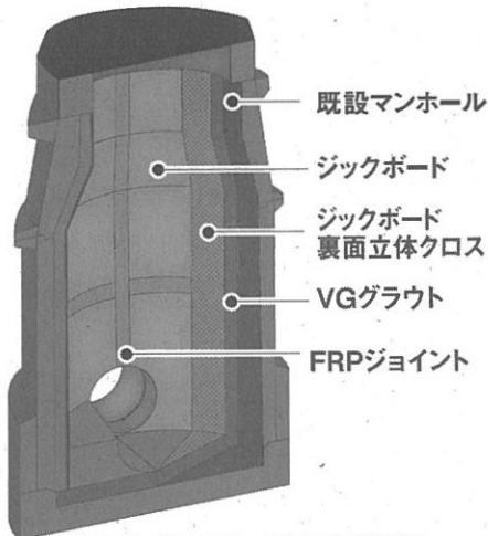
図-1 ジックボードVG工法断面図
