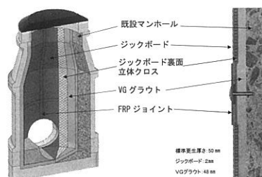
ジックボードVG工法の構成
